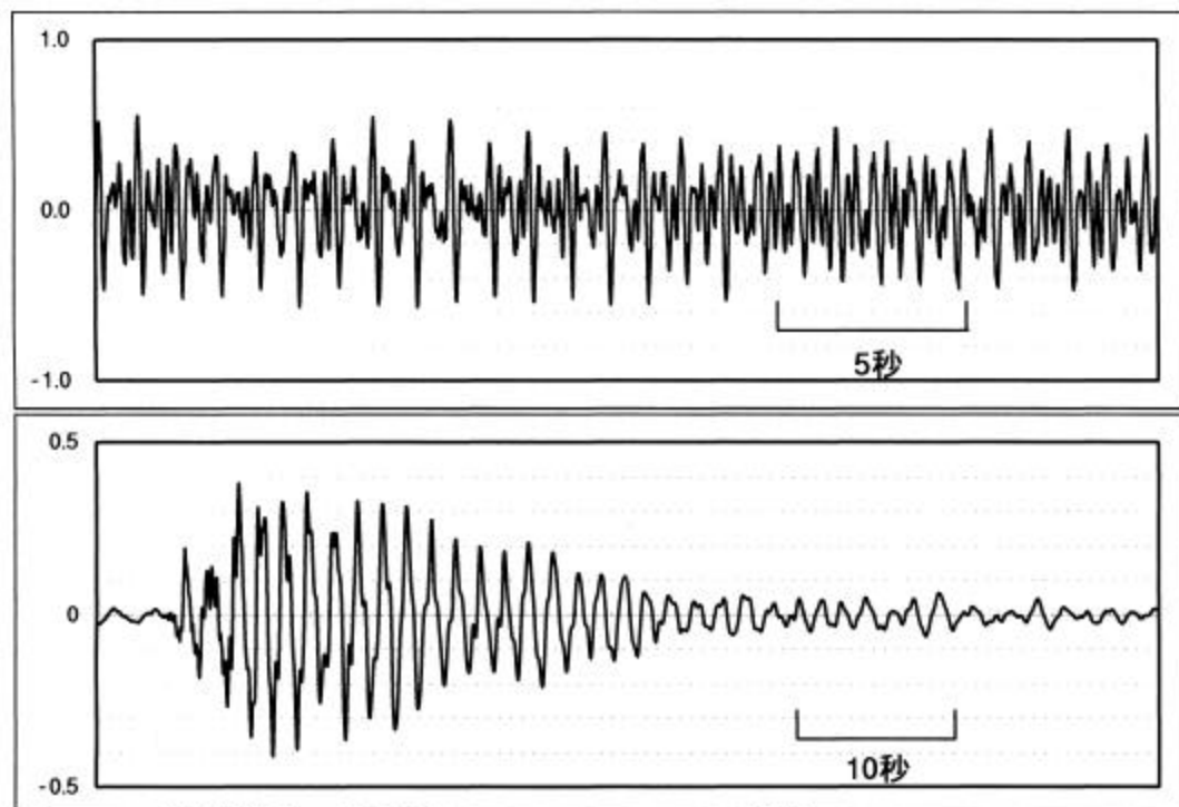
図1 連続微動の波形例(1991/6/19 06:30; NS成分) 図2 monocronicな波形の例(1998/1/27 19:27; NS成分) 縦軸の単位はmkine
