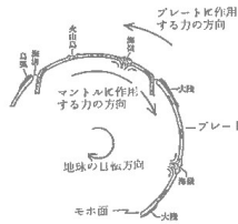
図-5. 海洋膨張大および大陸移動の模式図(上田 1971を参考に作成)
