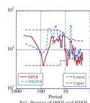
Fig.1. Spectra of DPOI and KDOI.
